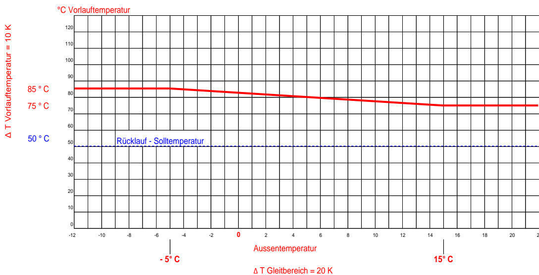
Abbildung 1: Netzvorlauftemperatur \theta_{VN} in Abhängigkeit von der Außentemperatur \theta_A ; prinzipieller Verlauf der gleitend-konstanten Fahrweise
