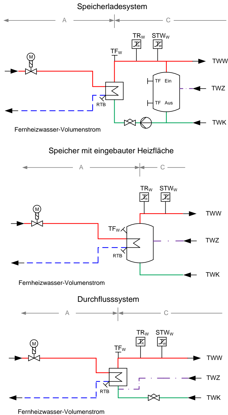
Abbildung 13: Hauszentrale-Trinkwassererwärmung Prinzipschaltbilder für den direkten Anschluss ohne Beimischregelung
