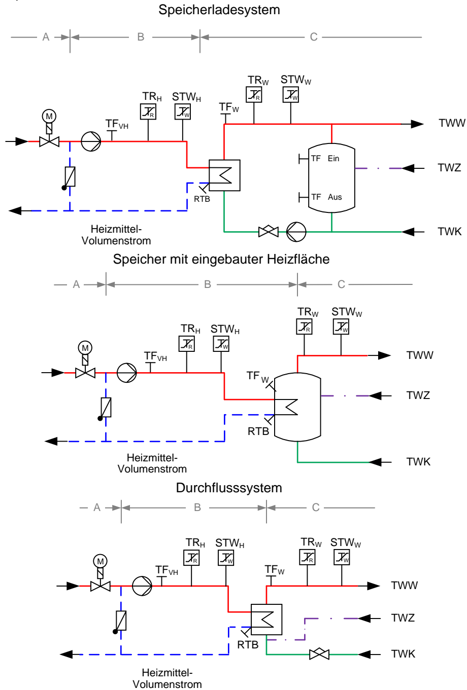
Abbildung 14: Hauszentrale-Trinkwassererwärmung Prinzipschaltbilder für den direkten Anschluss mit Beimischregelung
