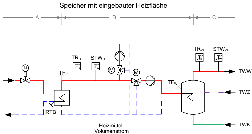
Abbildung 15: Hauszentrale-Trinkwassererwärmung Prinzipialschaltbild für den indirekten Anschluss
