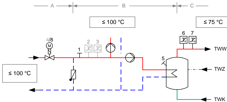
Abbildung zur Tabelle 11: Erforderliche sicherheitstechnische Ausrüstung nach Zeile 2; grau dargestellte Komponenten nicht erforderlich
