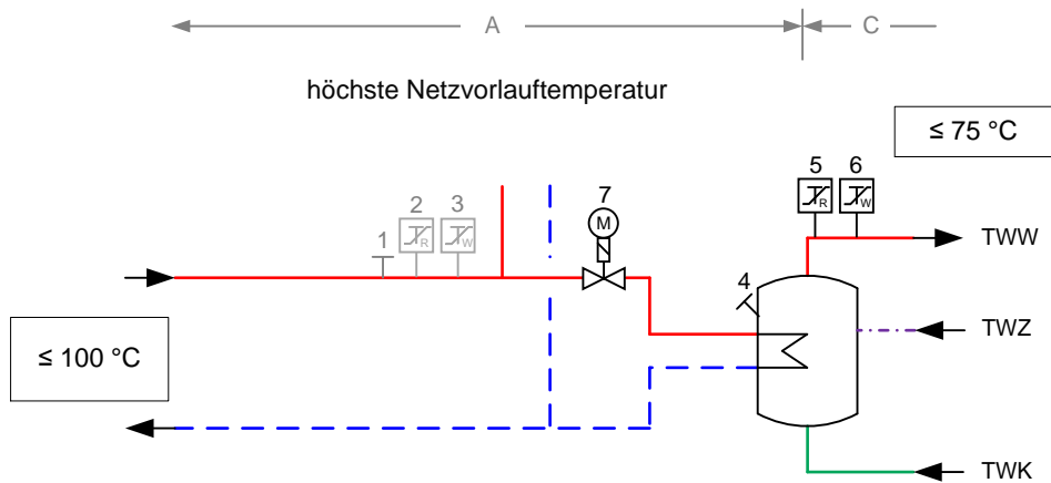
Abbildung zur Tabelle 9: Erforderliche sicherheitstechnische Ausrüstung nach Zeile 1; grau dargestellte Komponenten nicht erforderlich
