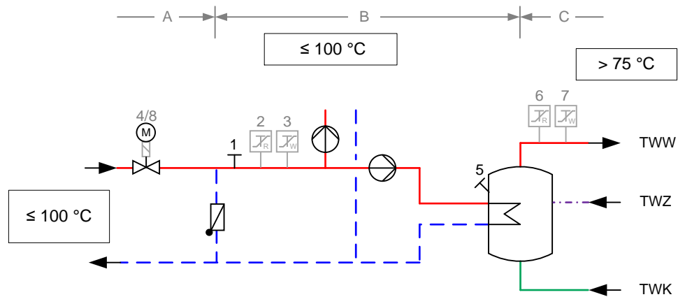
Abbildung zur Tabelle 13: Erforderliche sicherheitstechnische Ausrüstung nach Zeile 3; grau dargestellte Komponenten nicht erforderlich
