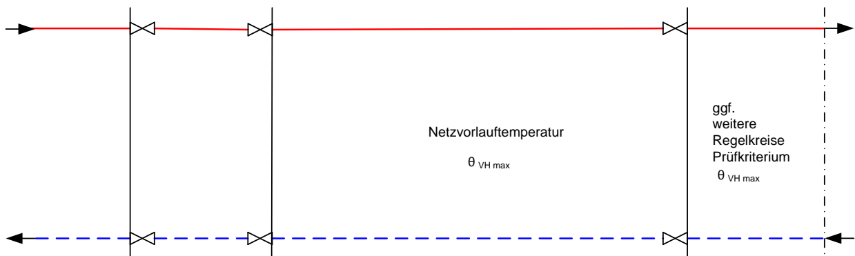
Abbildung zur Tabelle 5: keine sicherheitstechnische Ausrüstung erforderlich
