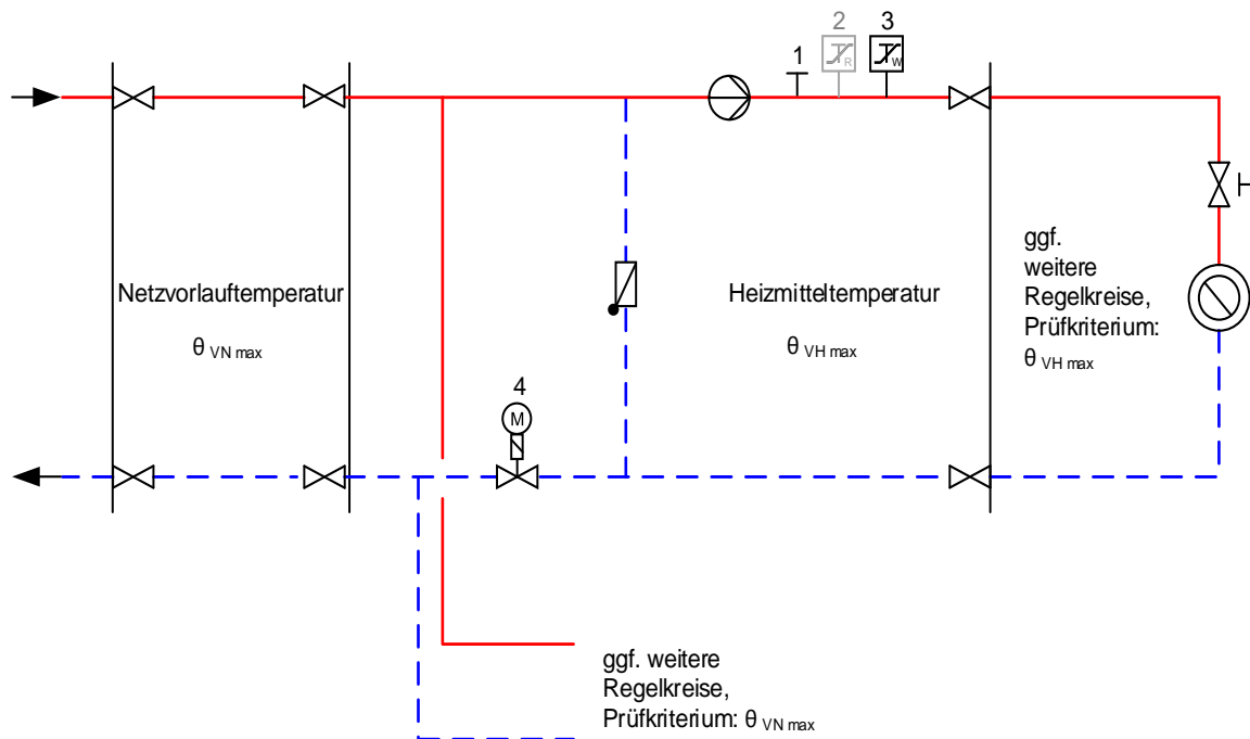
Abbildung zur Tabelle 2: Erforderliche sicherheitstechnische Ausrüstung nach Zeile 2; grau dargestellte Komponenten nicht erforderlich
