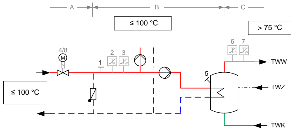
Abbildung zur Tabelle 11: Erforderliche sicherheitstechnische Ausrüstung nach Zeile 3; grau dargestellte Komponenten nicht erforderlich
