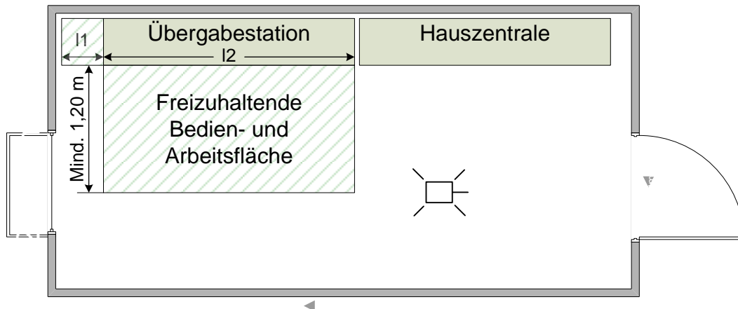
Abbildung 3: Hausanschlussraum
