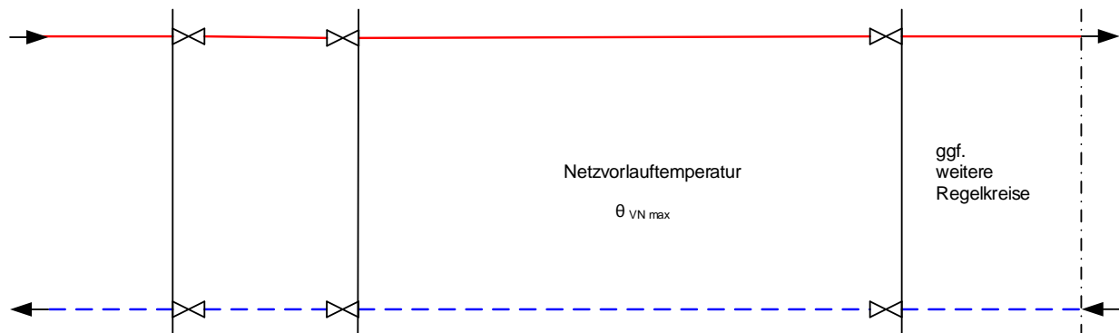
Abbildung zur Tabelle 1: Keine sicherheitstechnische Ausrüstung erforderlich
