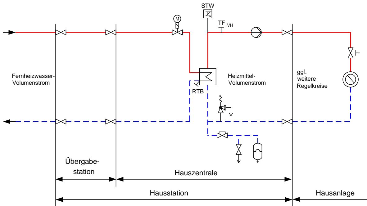
Abbildung 9: Hauszentrale-Raumheizung Prinzipialschaltbild für den indirekten Anschluss
