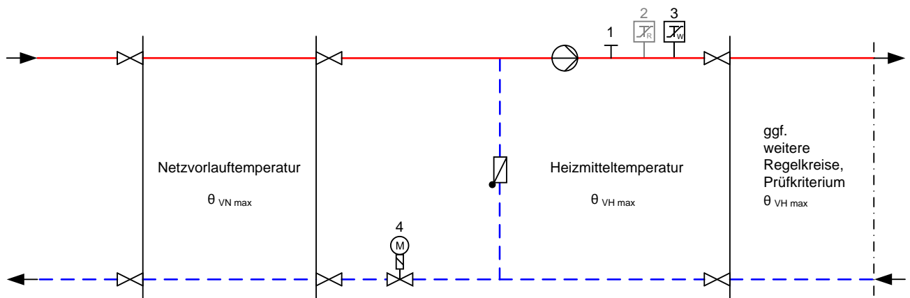
Abbildung zur Tabelle 6: Erforderliche sicherheitstechnische Ausrüstung nach Zeile 2; grau dargestellte Komponenten nicht erforderlich
