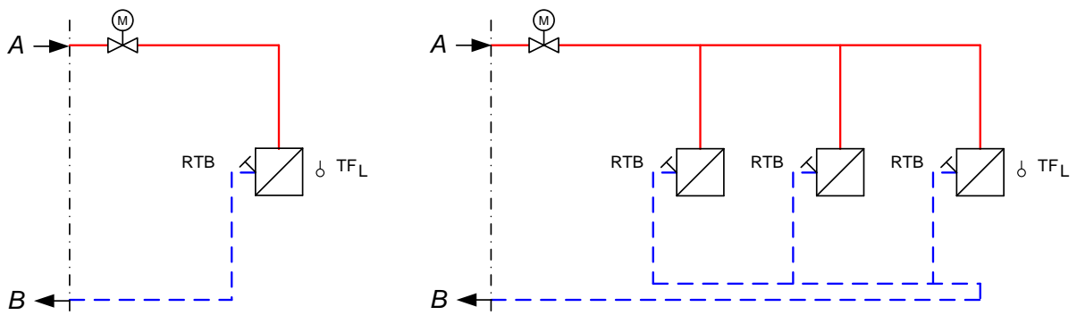
Abbildung 12: Hauszentrale-Raumluftheizung Prinzipschaltbilder für den indirekten Anschluss
